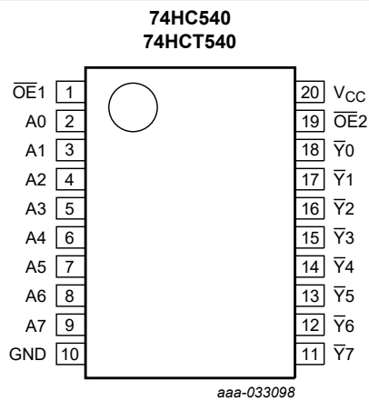
Fig. 6. Pin configuration SOT339-1 (SSOP20) and SOT360-1 (TSSOP20)
