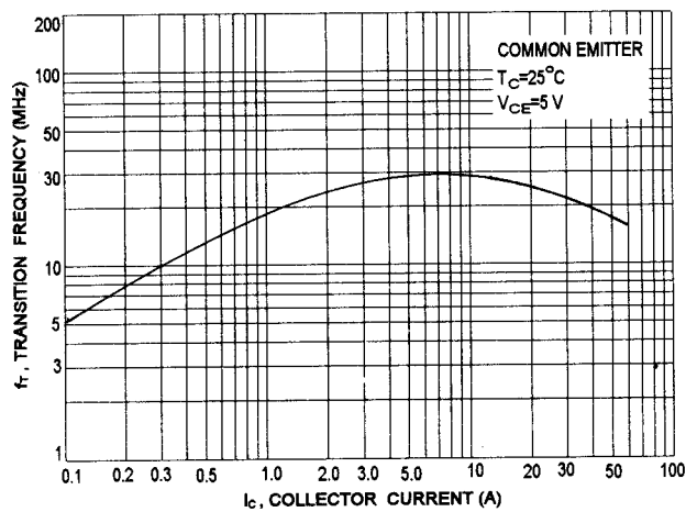
f_T - I_C
